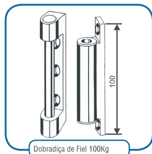
Dobradiça de Fiel Peso Máximo por folha 100kg
