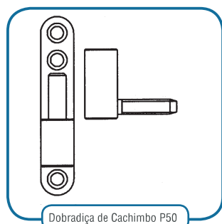
Dobradiça de Cachimbo Peso Máximo 50kg Parafusos Visíveis
