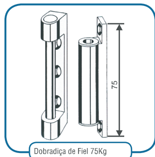
Dobradiça de Fiel Peso Máximo por folha 75kg
